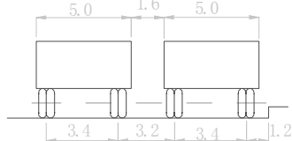
110t 汽车横向布置
