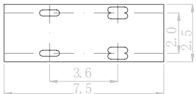
30t 汽车平面尺寸
