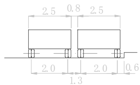
30t 汽车横向布置
