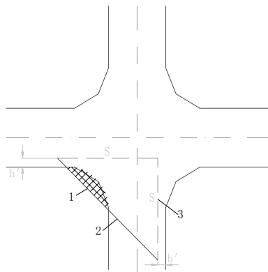
附图 4.3 交叉口视距图
