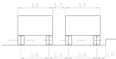
80t 汽车横向布置
