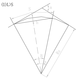
附图 4.1 不设回旋曲线时横净距计算图
