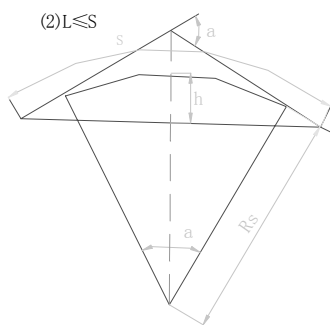
附图 4.1 不设回旋曲线时横净距计算图
