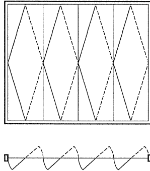
图 80 垂直中轴百叶窗
