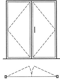
图 16 右开双扇内平开门
