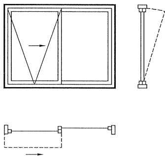
图73 右推拉下悬窗
