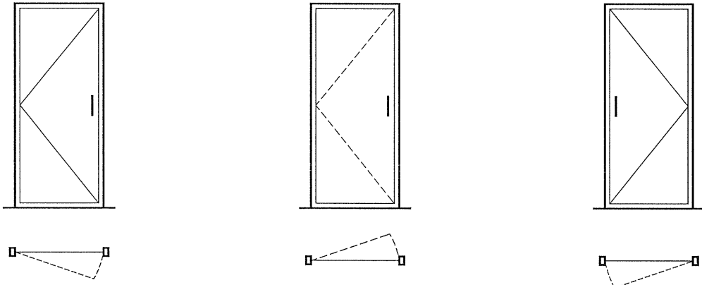
图5 左开[单扇]外平开门
