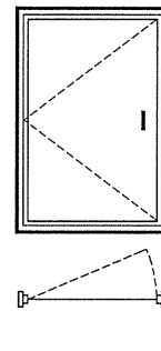
图 49 左开单扇外平开窗
