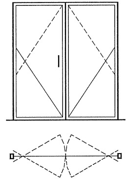
图 19 左开双扇双向地弹簧门
