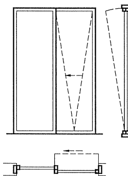
图 36 左推拉下悬门
