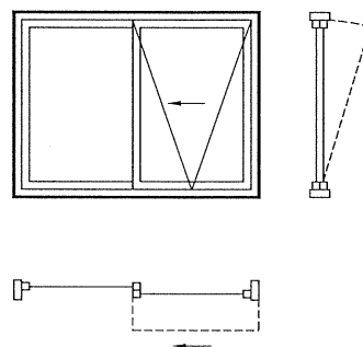
图74 左推拉下悬窗
