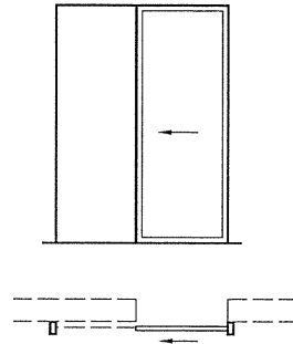
图 21 墙外单扇左推拉门
