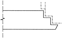
图 3 双企口扇
