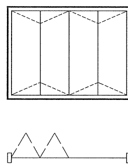
图77 折叠推拉窗
