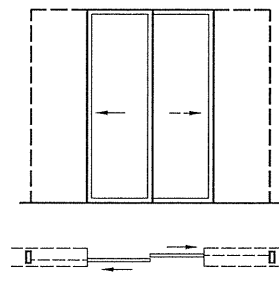
图 31 墙中左外扇推拉门
