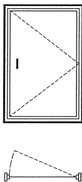
图 50 右开单扇外平开窗
