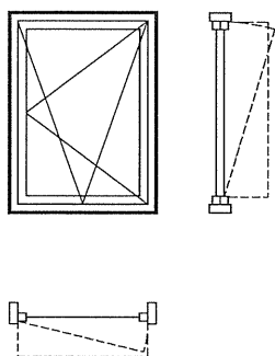
图75 左开内平开下悬窗
