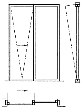
图 35 右推拉下悬门
