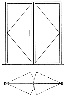
图 17 左开双扇双向弹簧门
