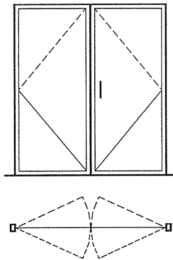
图 18 右开双扇双向弹簧门
