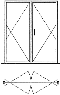
图 20 右开双扇双向地弹簧门
