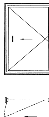
图 52 右开单扇滑轴内平开窗
