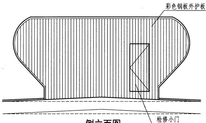
侧立面图
