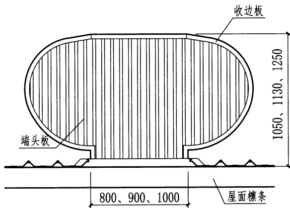
立面图
