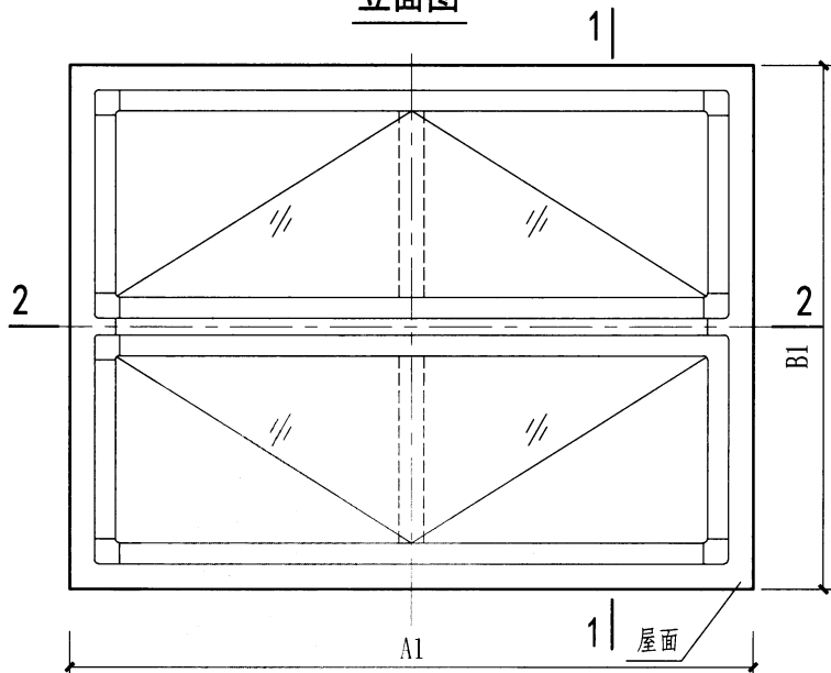
平面图
