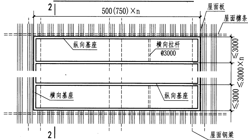
2 | MCW1、2型纵向通风天窗基座平面布置图
