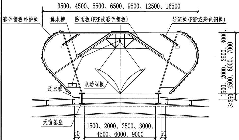
剖面图
