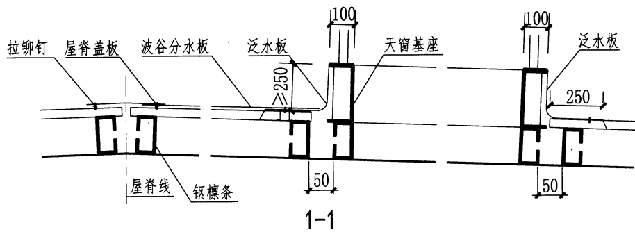
点支撑天窗基座示意图一
