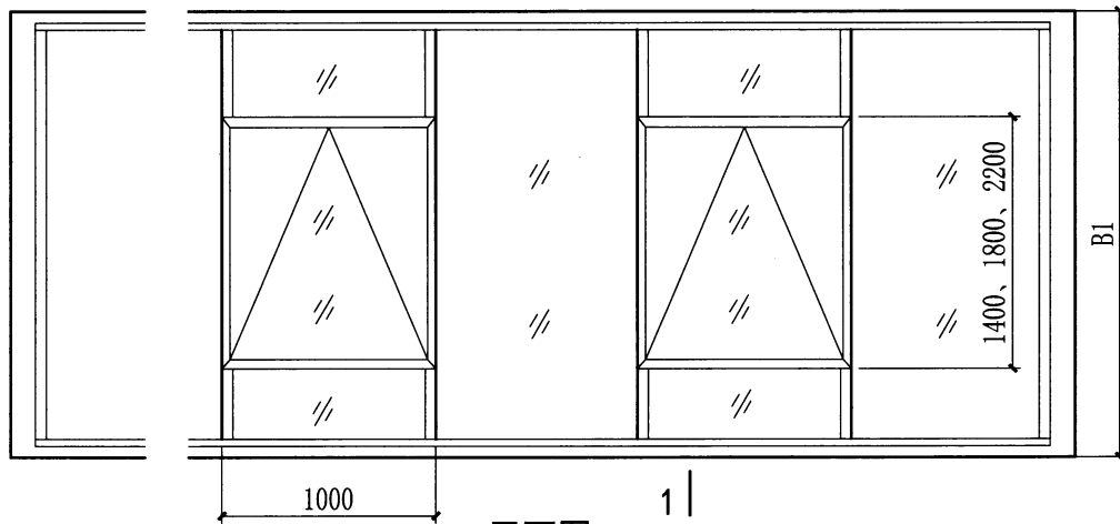
平面图
