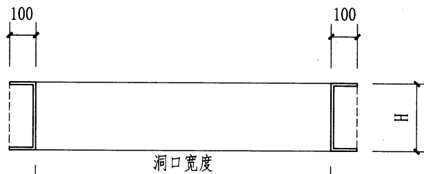
2-2剖面图 (用于横向通风天窗)
