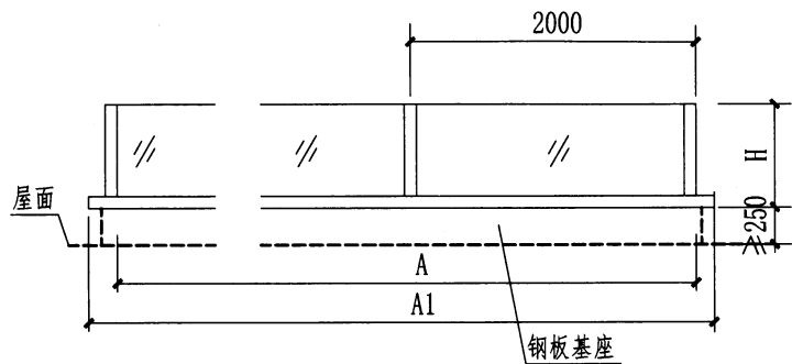
立面图
