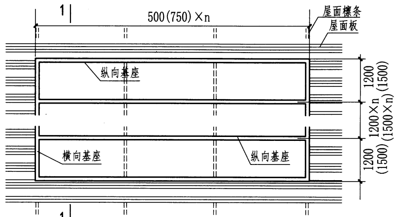
1 | MCW1、2型横向通风天窗基座平面布置图
