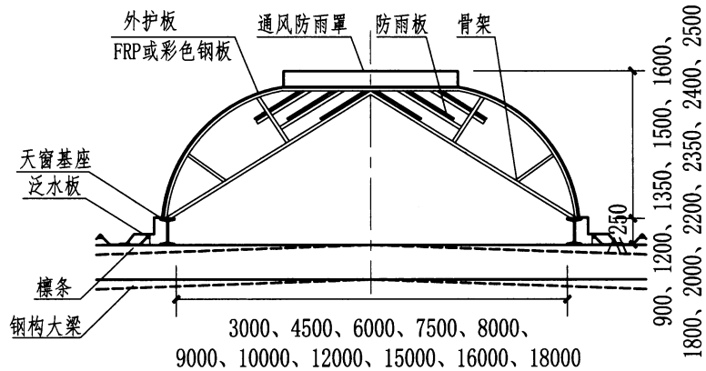
剖面图
