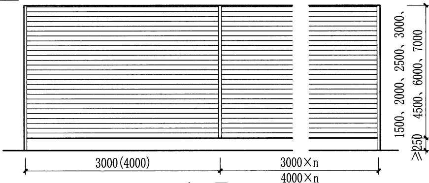
立面图
