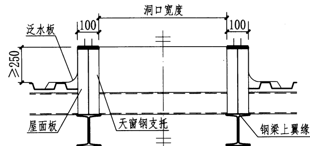
点支撑天窗基座示意图二
