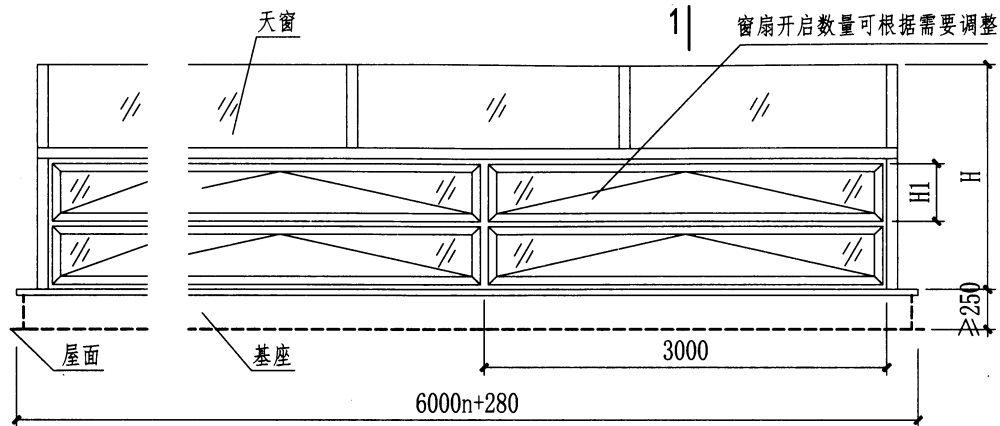
立面图 1
