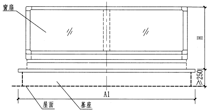
立面图
