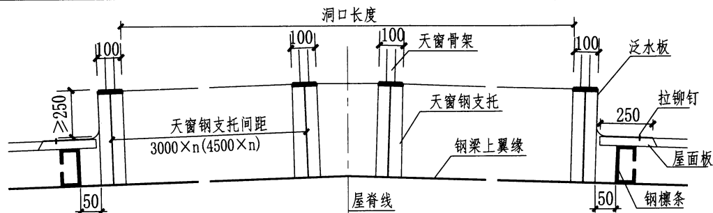
点支撑天窗基座示意图一
