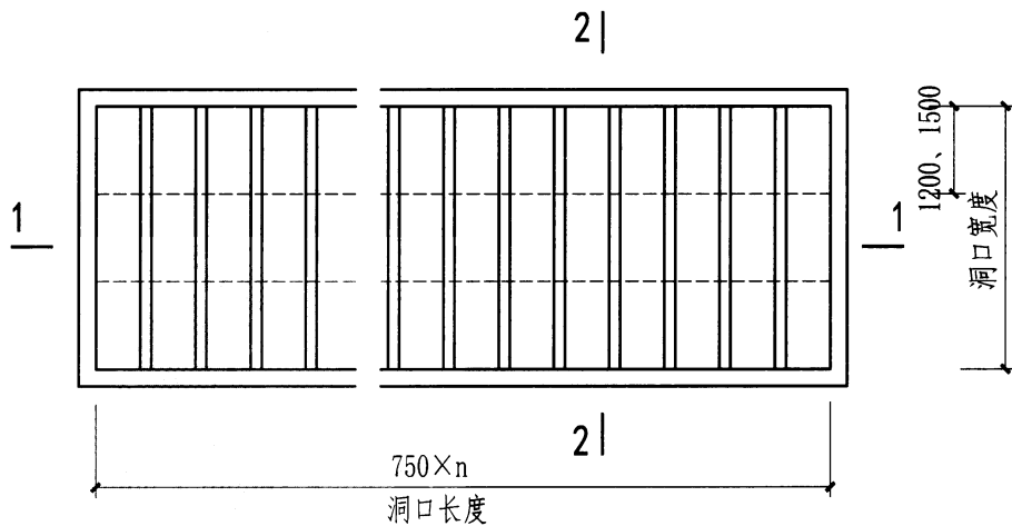
平面图
