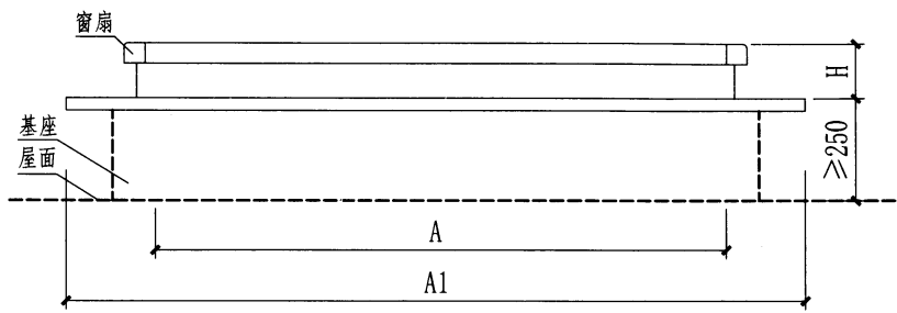
立面图
