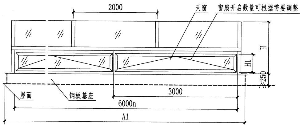
立面图
