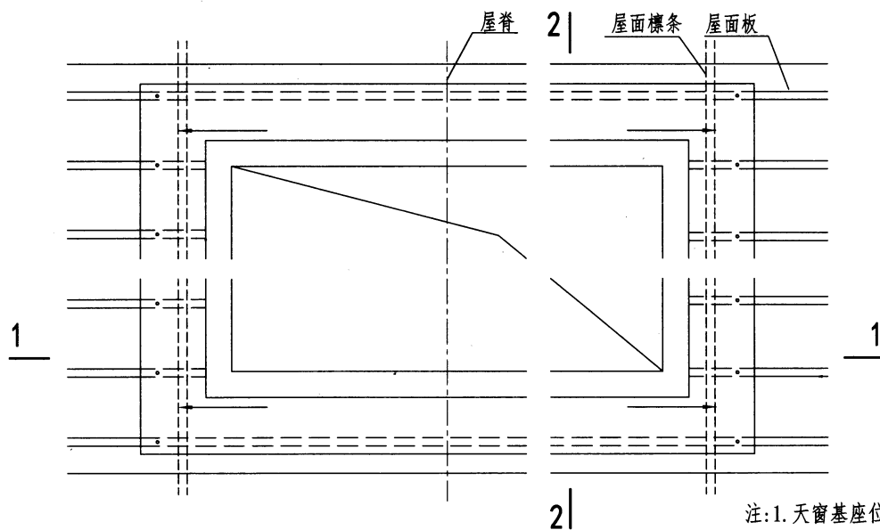
天窗基座洞口平面图
