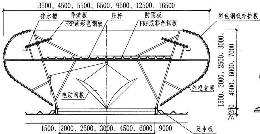
剖面图
