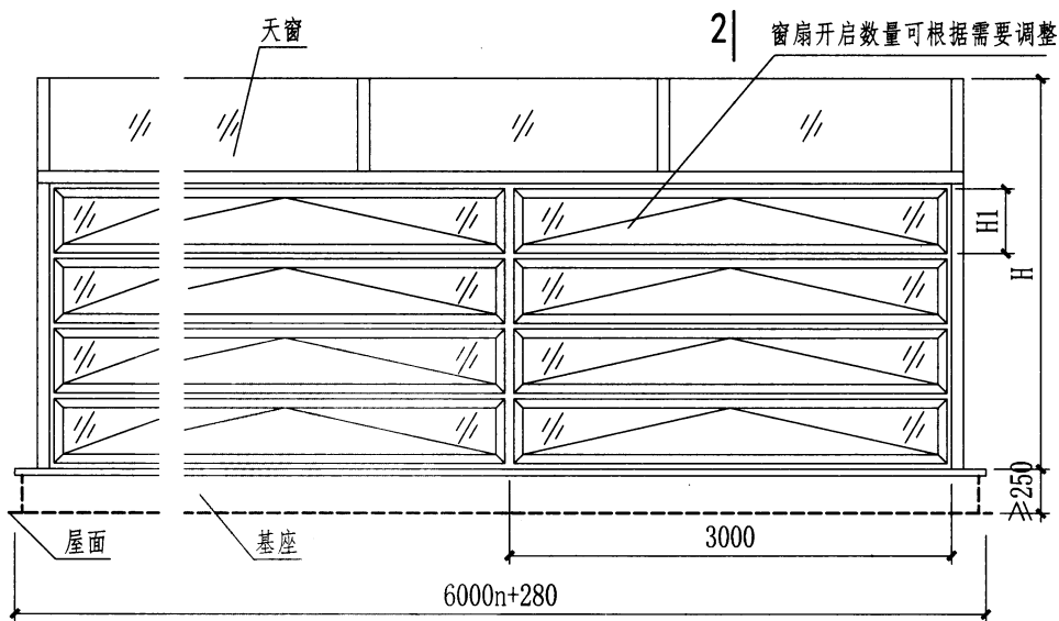
立面图 2
