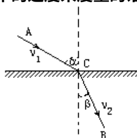
图 21 —最短时间原理
